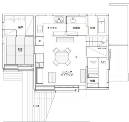
1F平面図
