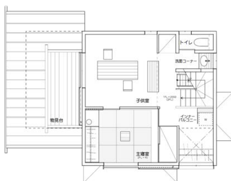
2F平面図
