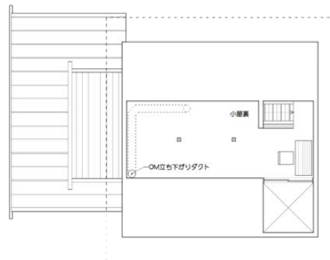
ロフト平面図
